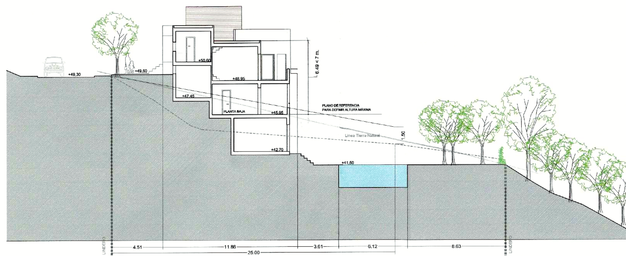
SECCIÓN 2-2
