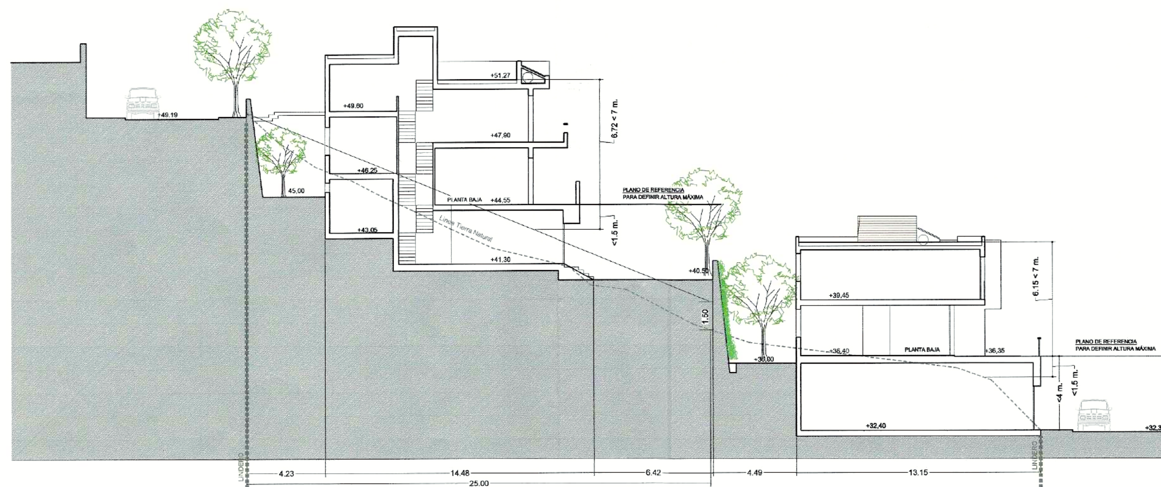
SECCIÓN 3-3
