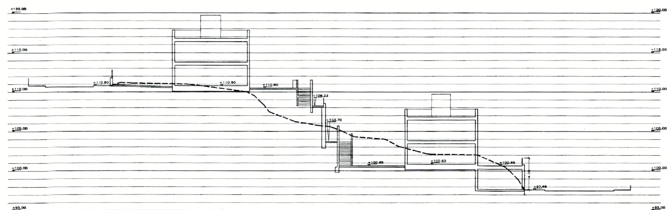
PERFIL DE LAS PARCELAS 31 Y 16
