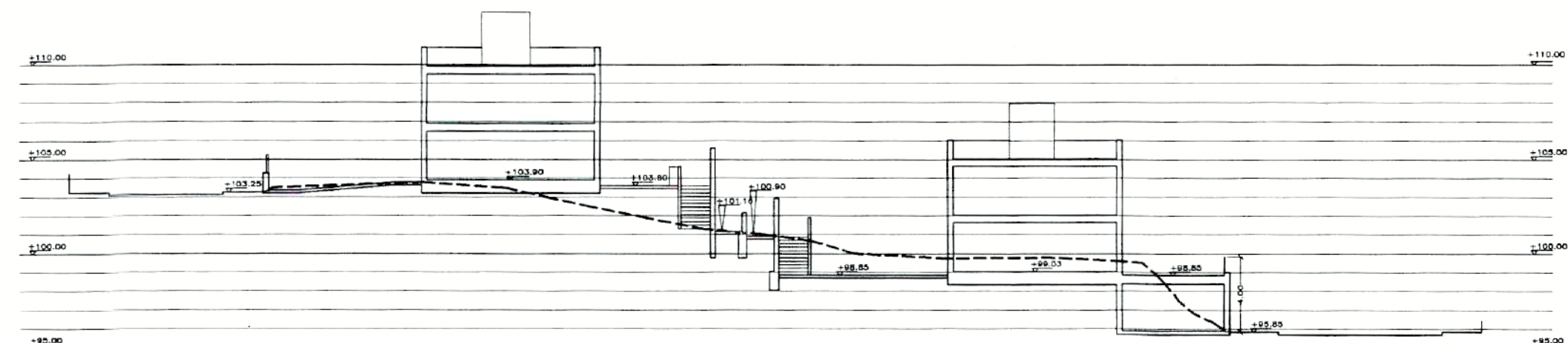
PERFIL DE LAS PARCELAS 3 Y 44
