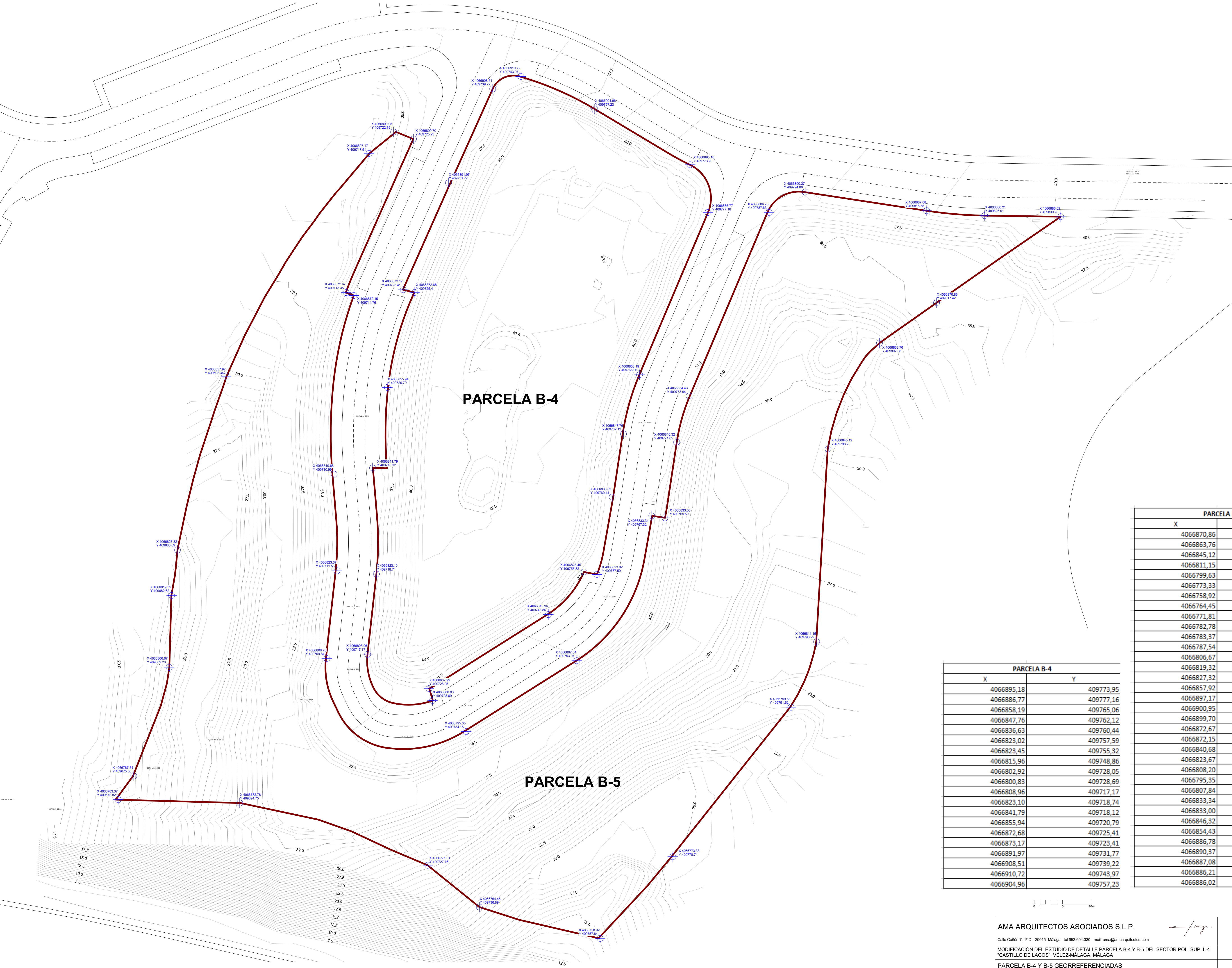
PARCELA B-4 Y B-5 GERREFERENCIADAS ESCALA: 1 : 300
