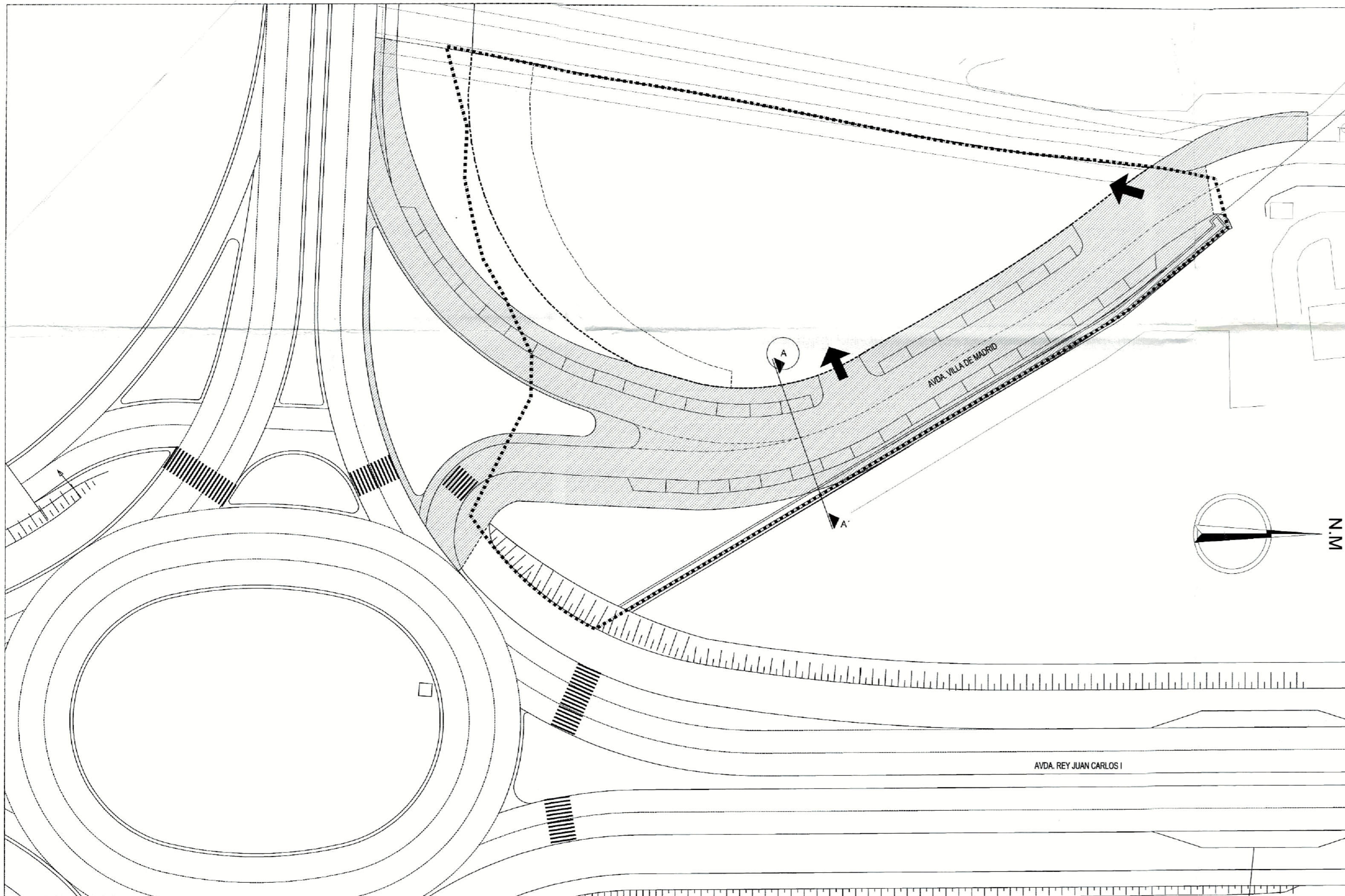
RED VIARIA ESCALA 1:500
