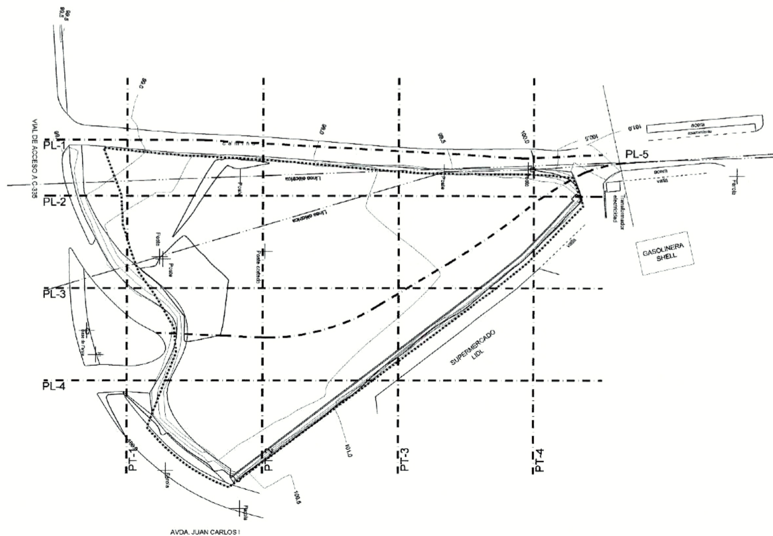
PLANO GUÍA DE PERFILES
