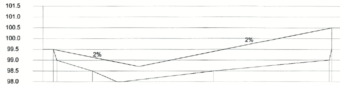
PERFIL PL-2. PERFIL POR PARCELA
