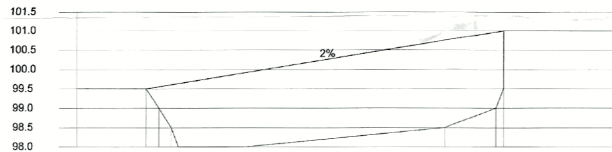
PERFIL PL-3. PERFIL POR PARCELA
