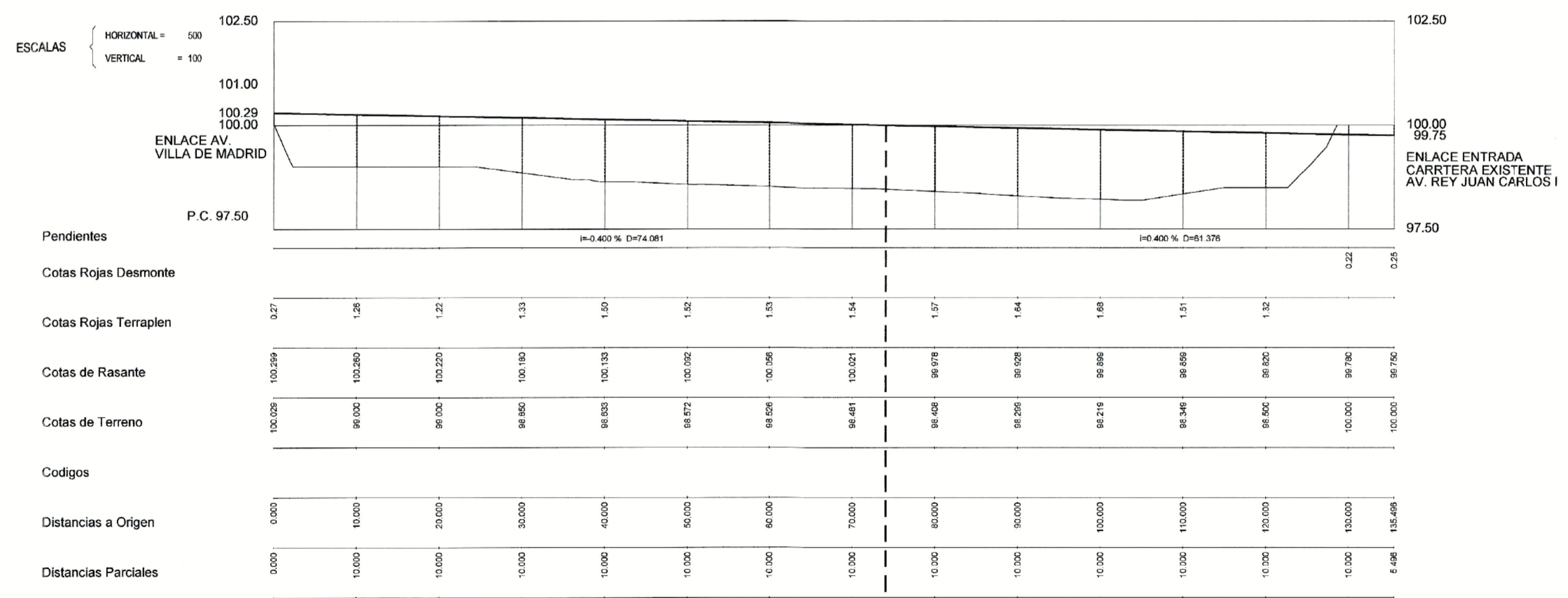
Perfil Longitudinal por Ramal de Entrada
