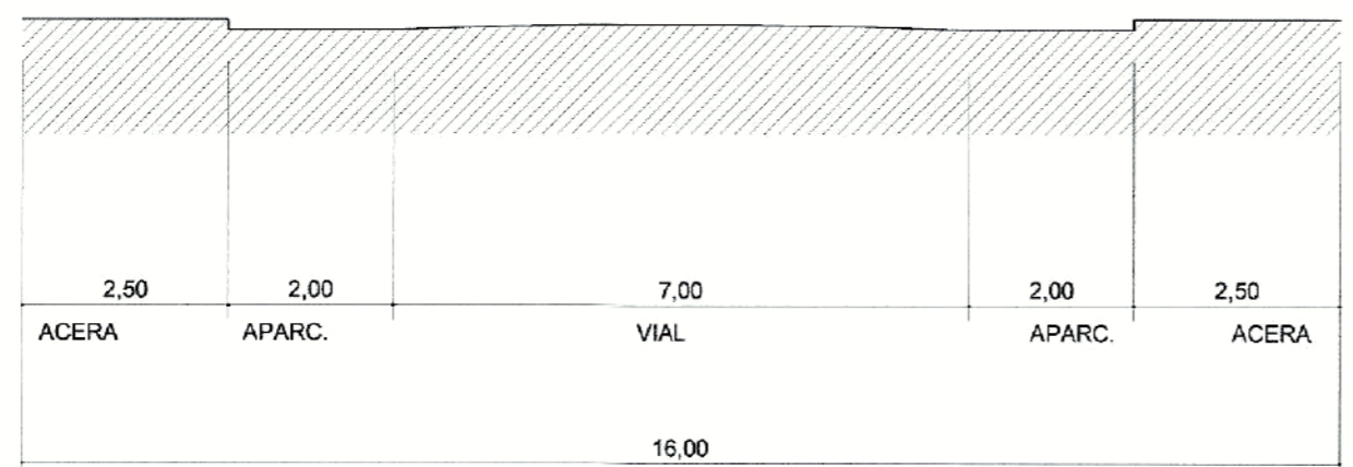
AVDA. VILLA DE MADRID SECCIÓN AA' ESCALA 1:100
